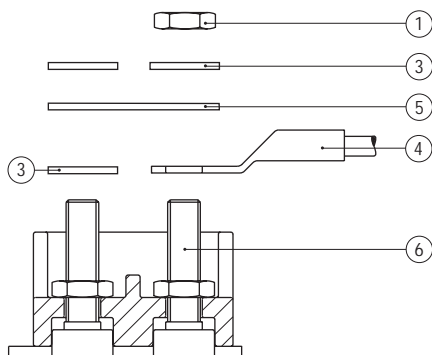
Fig. 1 - Sequenza di collegamento 56-80 (carcasa alluminio)
