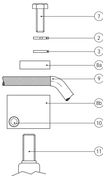
Fig. 3 - Sequenza di collegamento 280-315 (carcasa ghisa)
