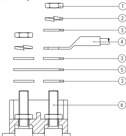
Fig. 2 - Sequenza di collegamento 63-250 (carcasa ghisa)
