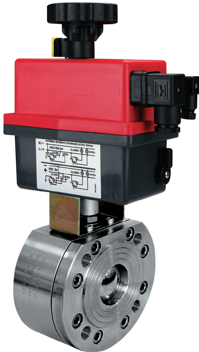
ATT. ELETTRICO (dal DN50 al DN100) EL 12-48 VDC / 15-48 VAC EH 80-240 VAC VDC
